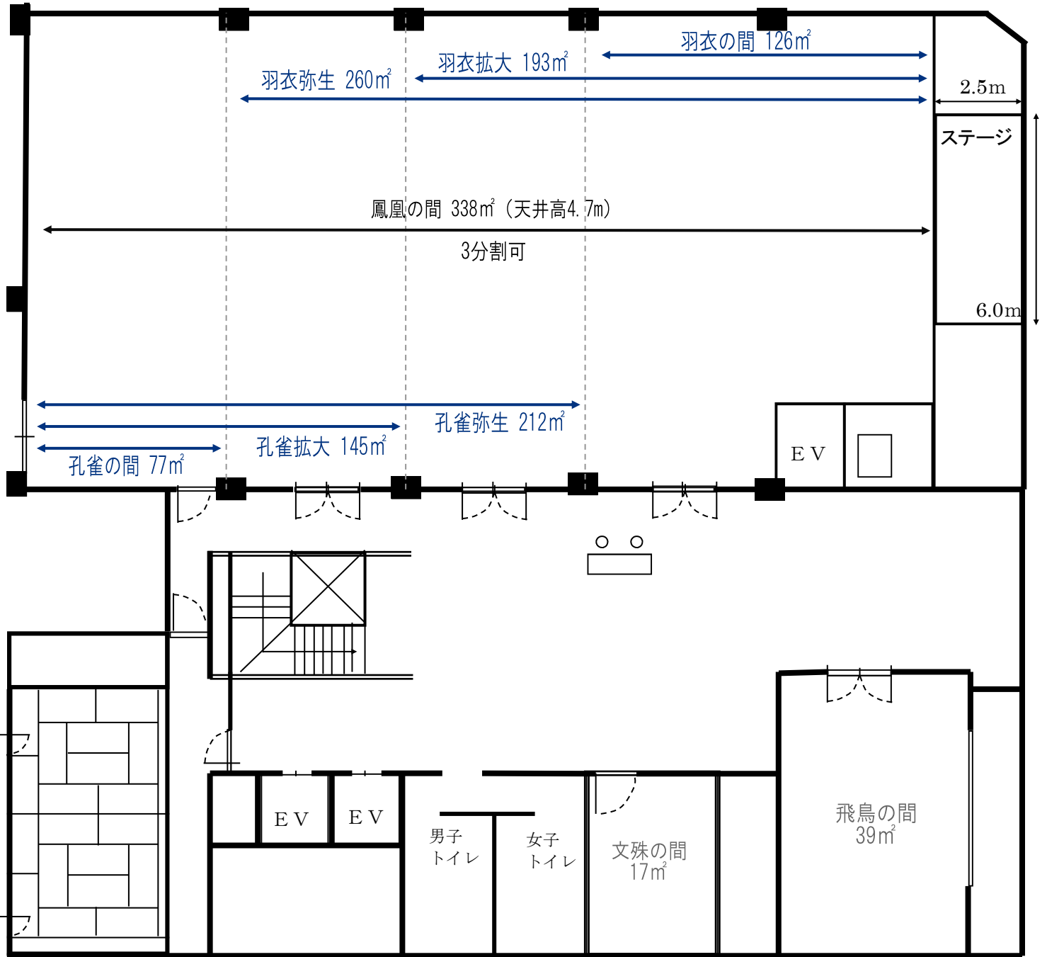
本館三階 平面図
